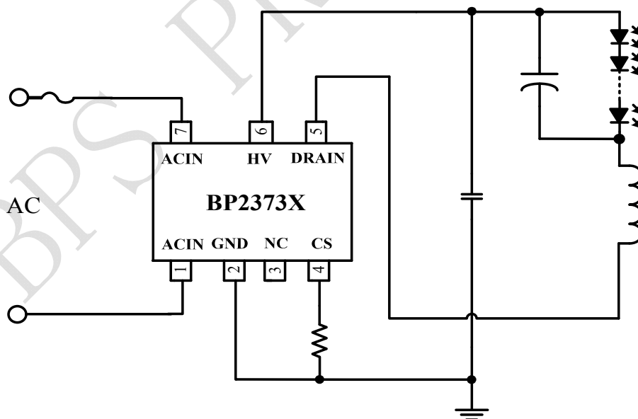
图 1 BP2373X 典型应用图
