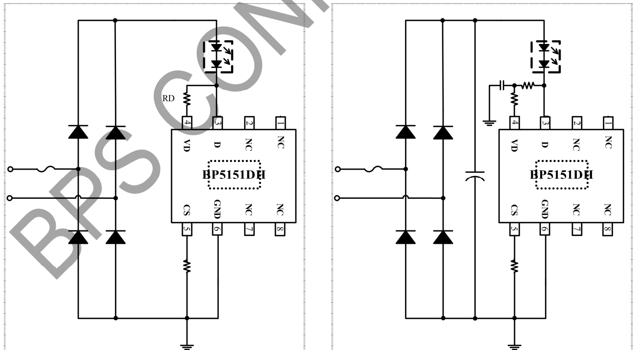
图 1 BP5151DH 典型应用图
