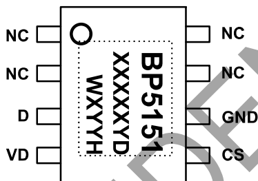
图 2 BP5151DH 管脚封装图
