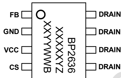
图 2 管脚封装图
