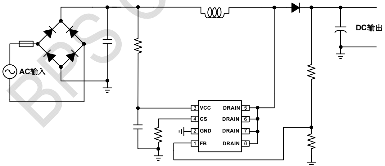
图 1 BP2636B 典型应用电路
